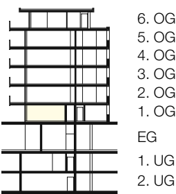
Schnitt
