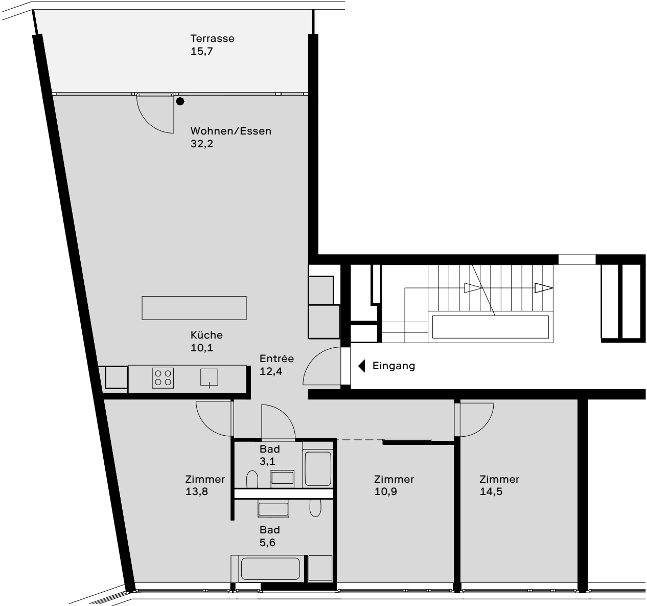
Grundriss
