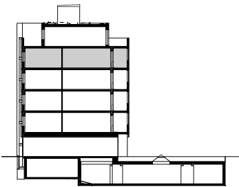
Schnitt
