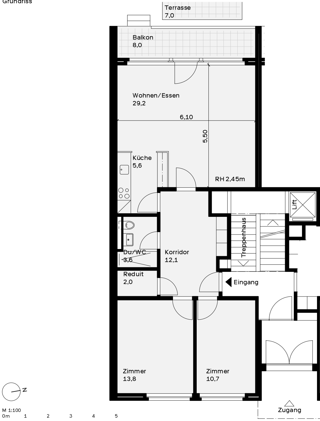
Grundriss
