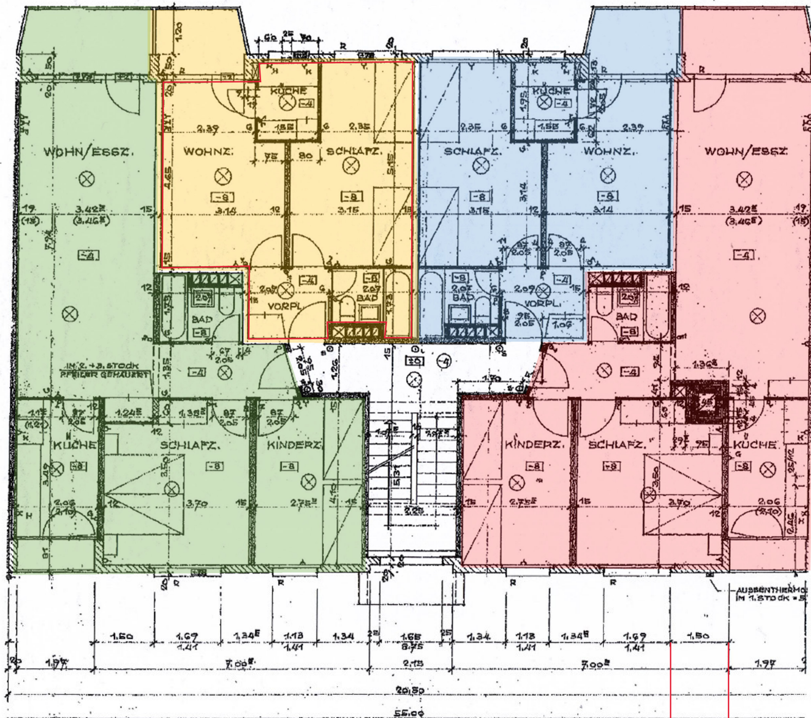
HAUS 9. GRUNDRISS ERDG. 1.-3. STOCK
