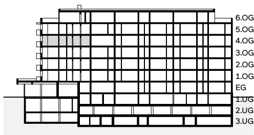
Schnitt
