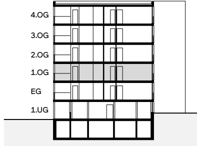
Schnitt
