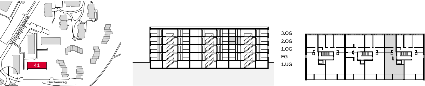
Situation Schnitt Übersicht Grundriss EG
