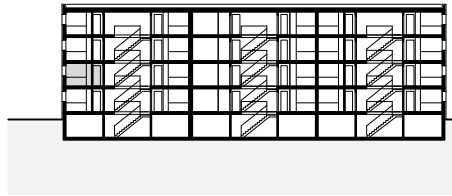
Schnitt
