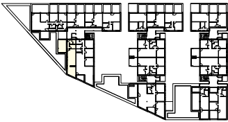
Übersicht 3. OG
