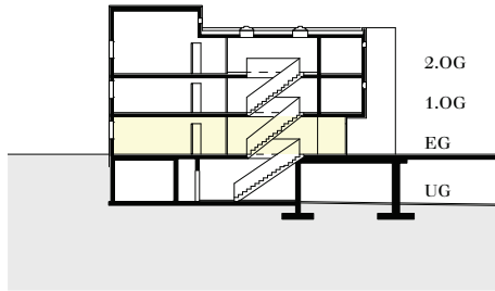
Schnitt
