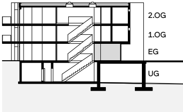
Schnitt
