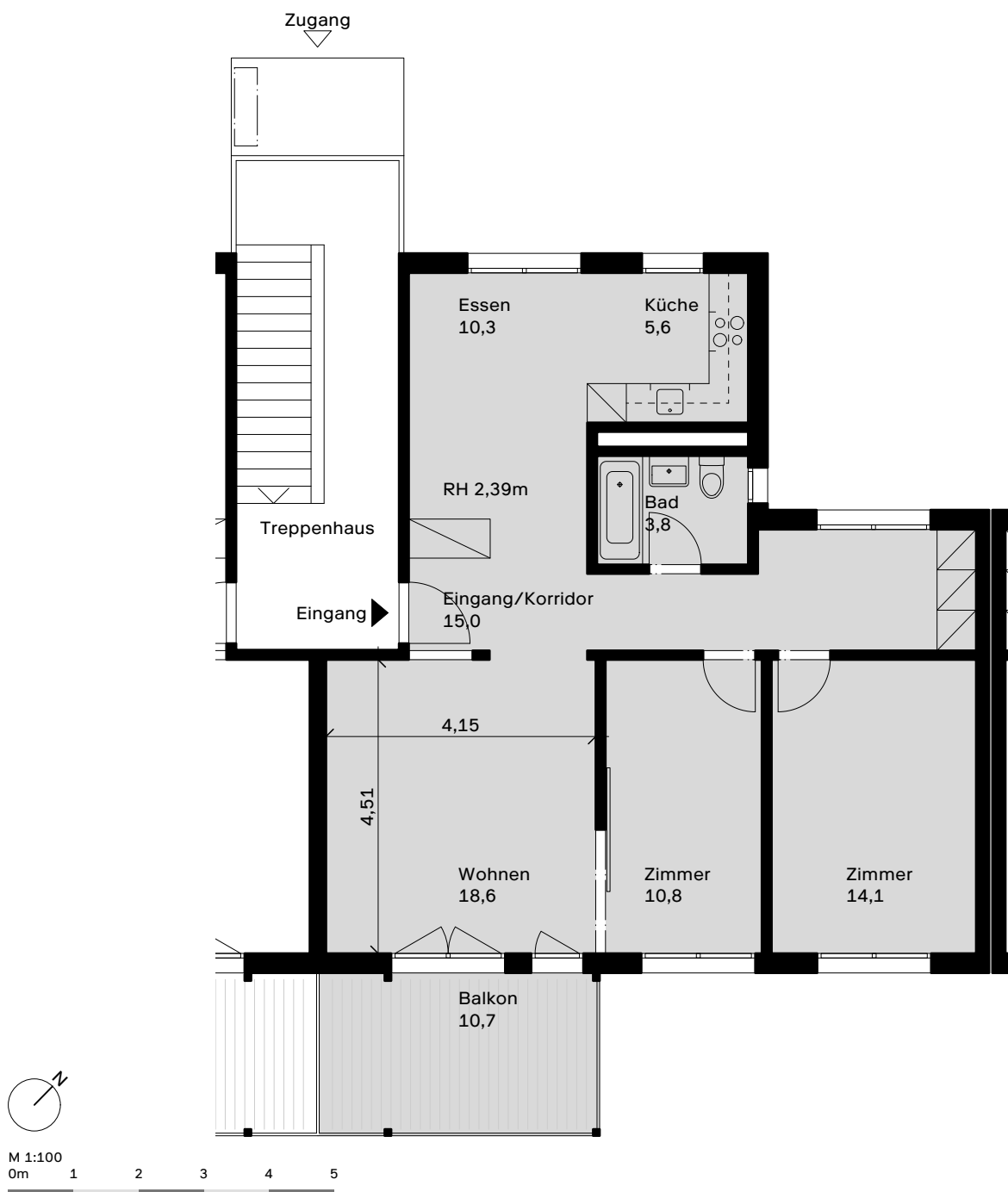
Grundriss
