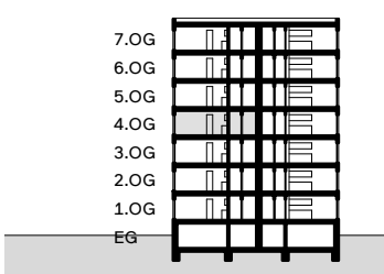
Schnitt
