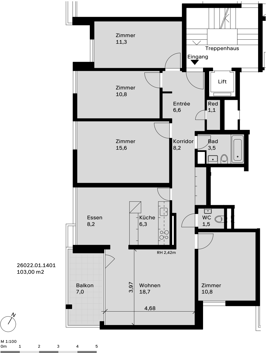
Grundriss
