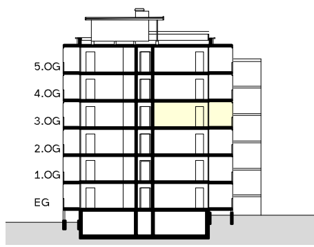
Schnitt
