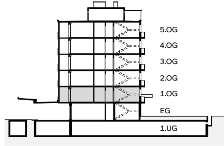
Schnitt
