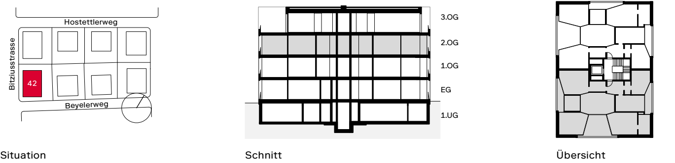
Grundriss
