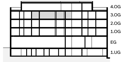
Schnitt
