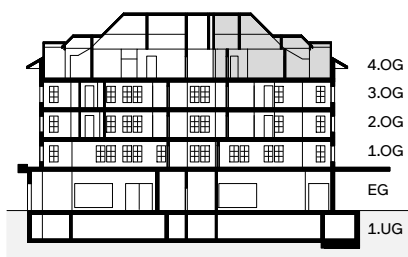
Schnitt
