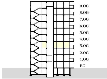
Schnitt
