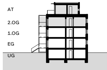
Schnitt
