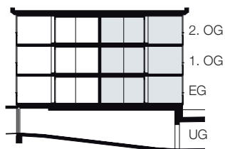
Schnitt
