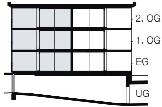
Schnitt
