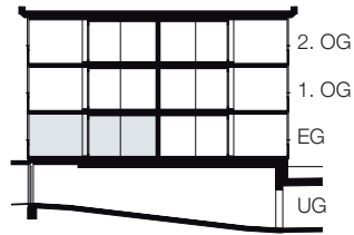
Schnitt
