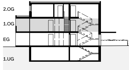
Schnitt
