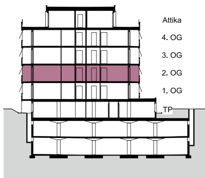
Schnitt
