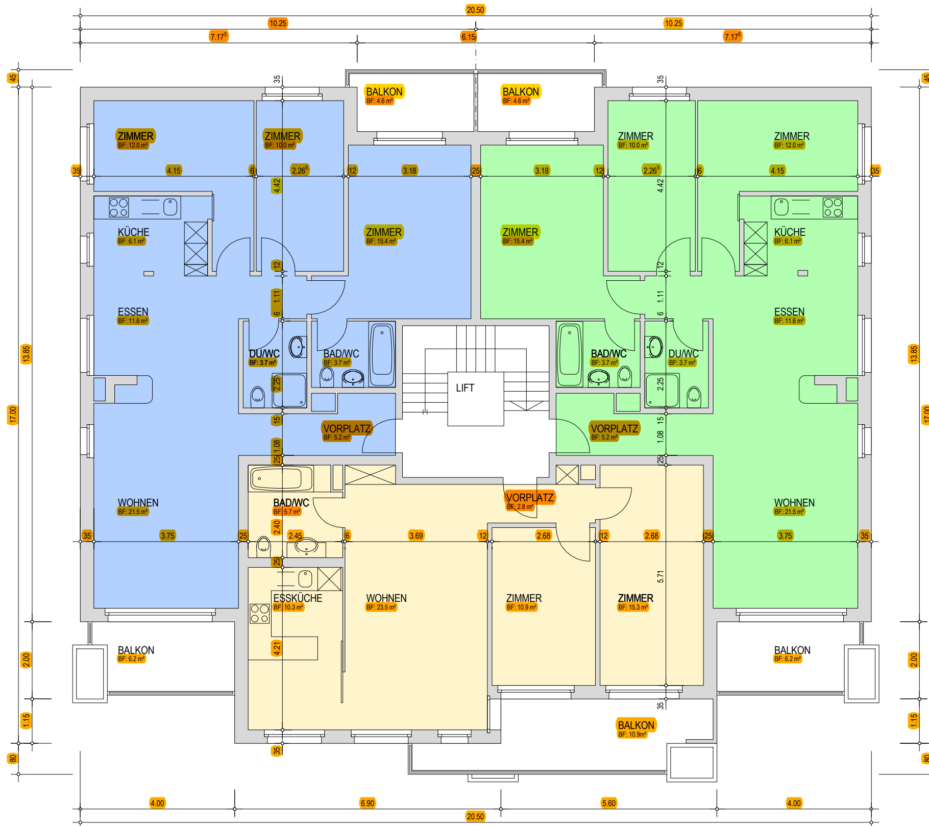
SOLOTHURNSTRASSE 67/67a/67b, LENGNAU 3 MEHRFAMILIENHÄUSER GRUNDRISS OBERGESCHOSS 1:100
