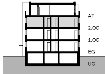
Schnitt
